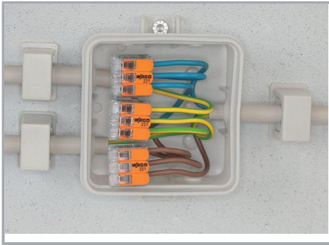
Verdrahtung feindrhtiger Leiter in Installationsdosen
